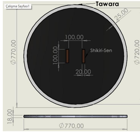
Şekil 1: Dohyo Ölçüleri
